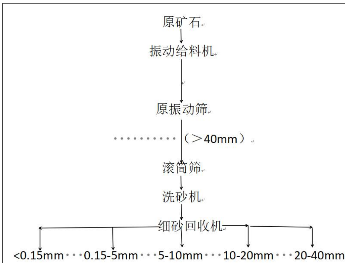
图 2-8 工艺流程图
