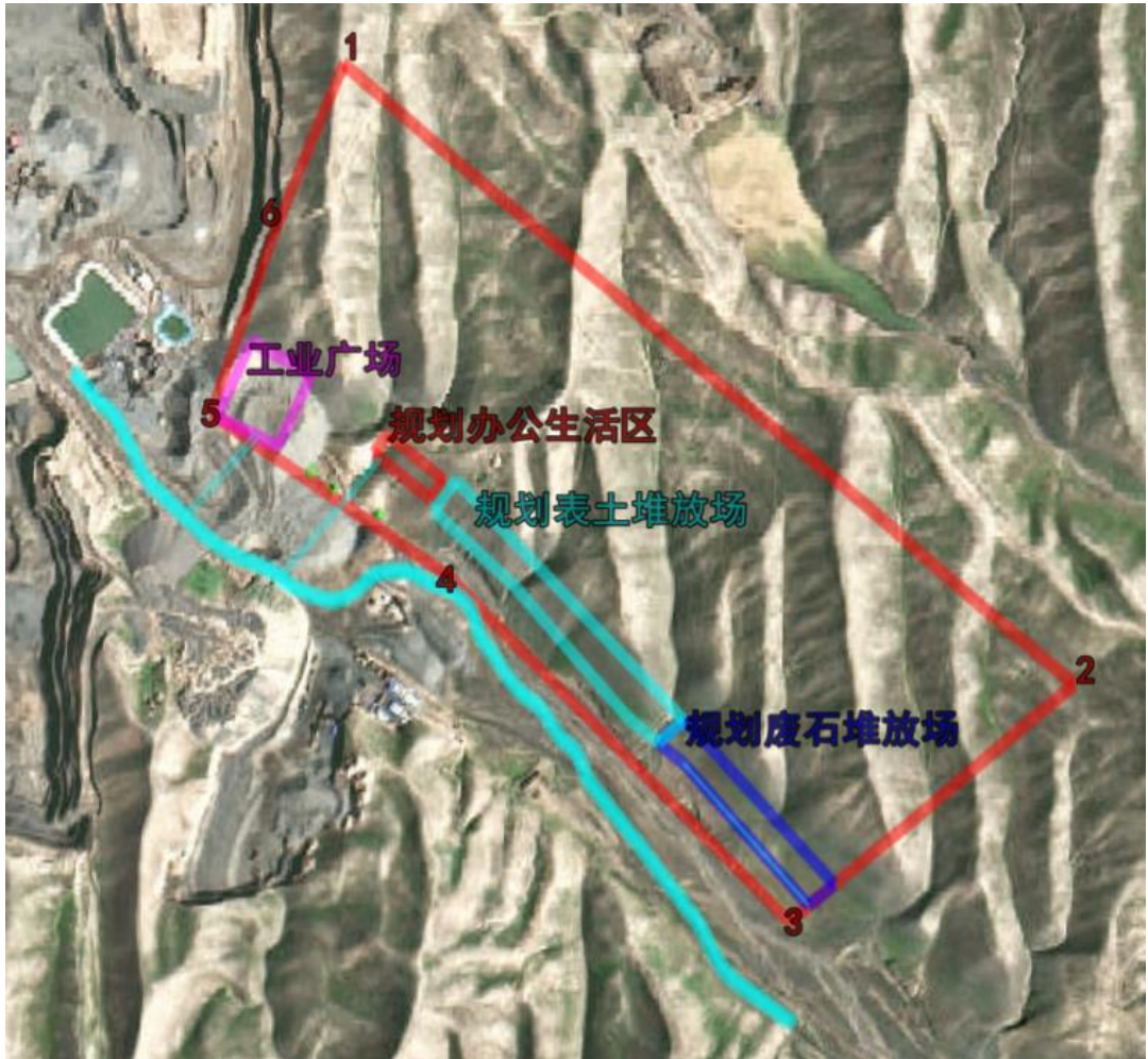
图 3-2 总平面布置图
