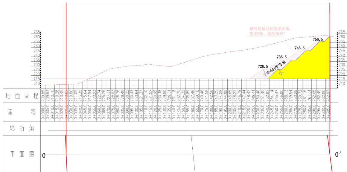
图 5-3 0-0' 复垦剖面图
